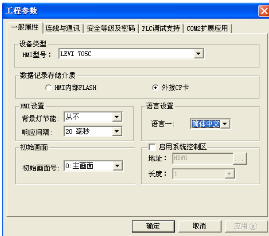
图 11-7 编译语言的配置
