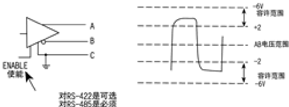
图 22-2 RS-422/RS-485 线定义
