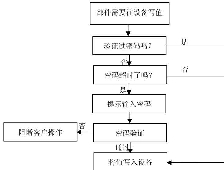
图 16-13 按键密码保护原理
